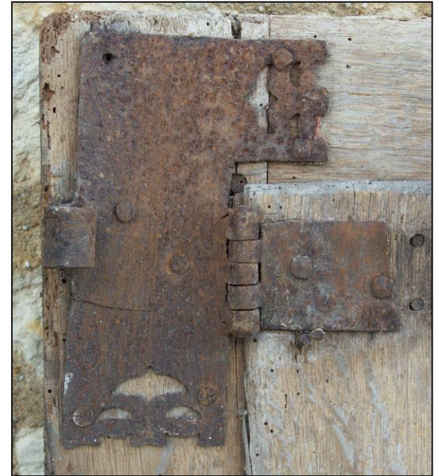
Fig. 1.3. Penture à charnière
