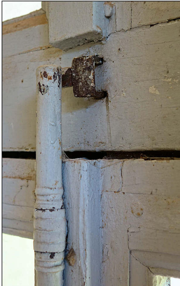
Fig. 5.2. Embase / crochet et gâche
