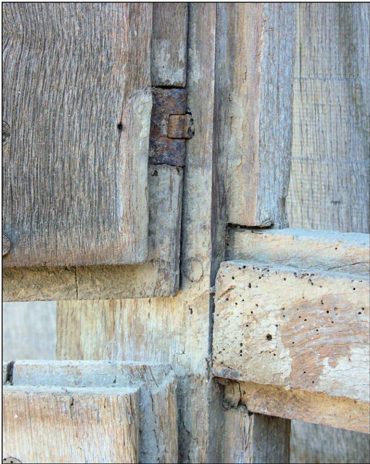
Fig. 2.3. Assemblage du croisillon / fiche à broche rivée
