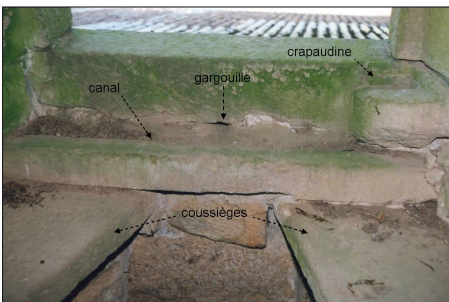
Fig. 2.7. Appui de la fenêtre
