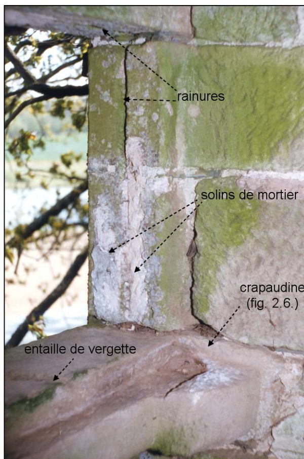
Fig. 2.5. Tableau droit / compartiment supérieur
