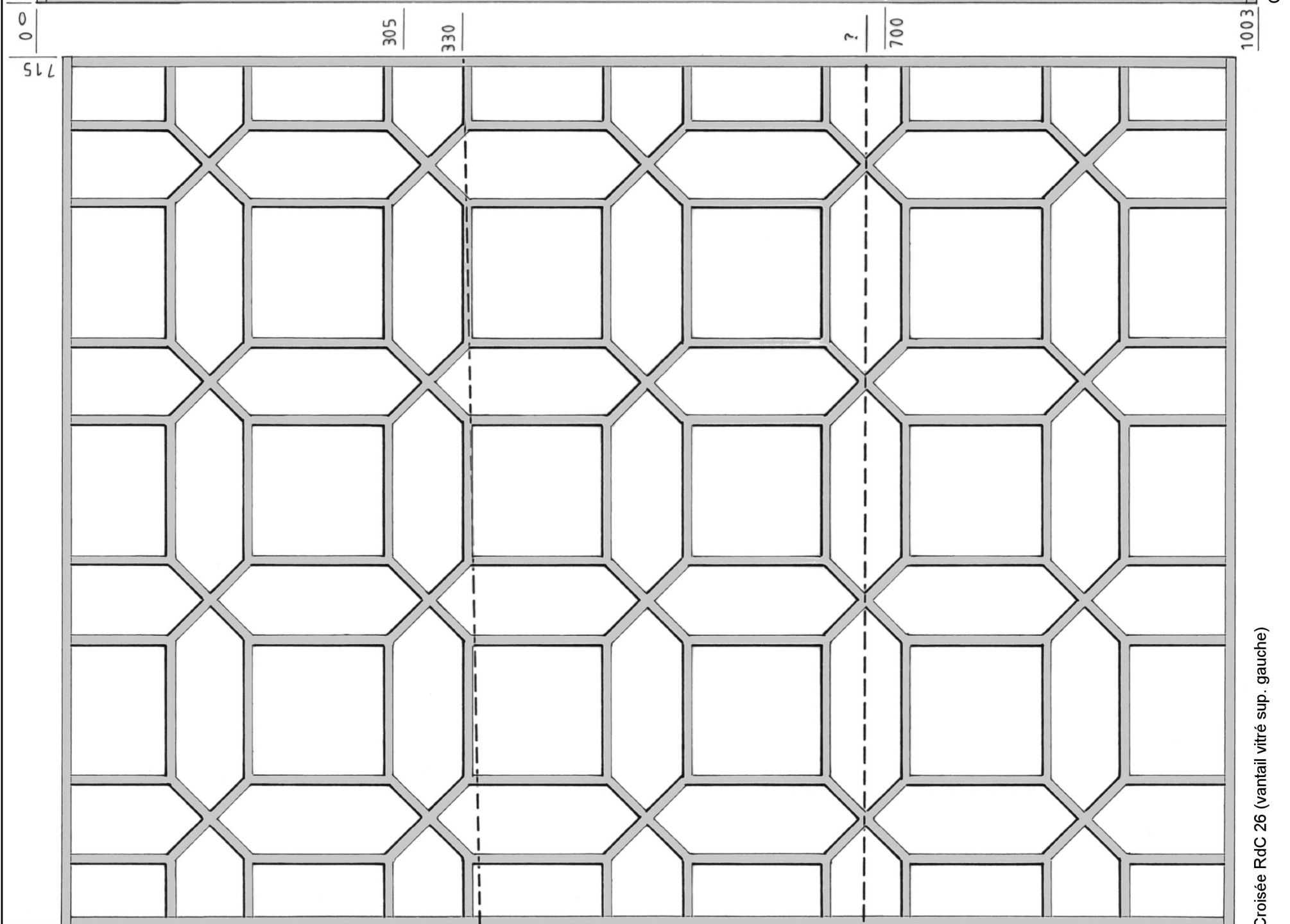
Croisée E 32 (vantail vitré inf. gauche)
