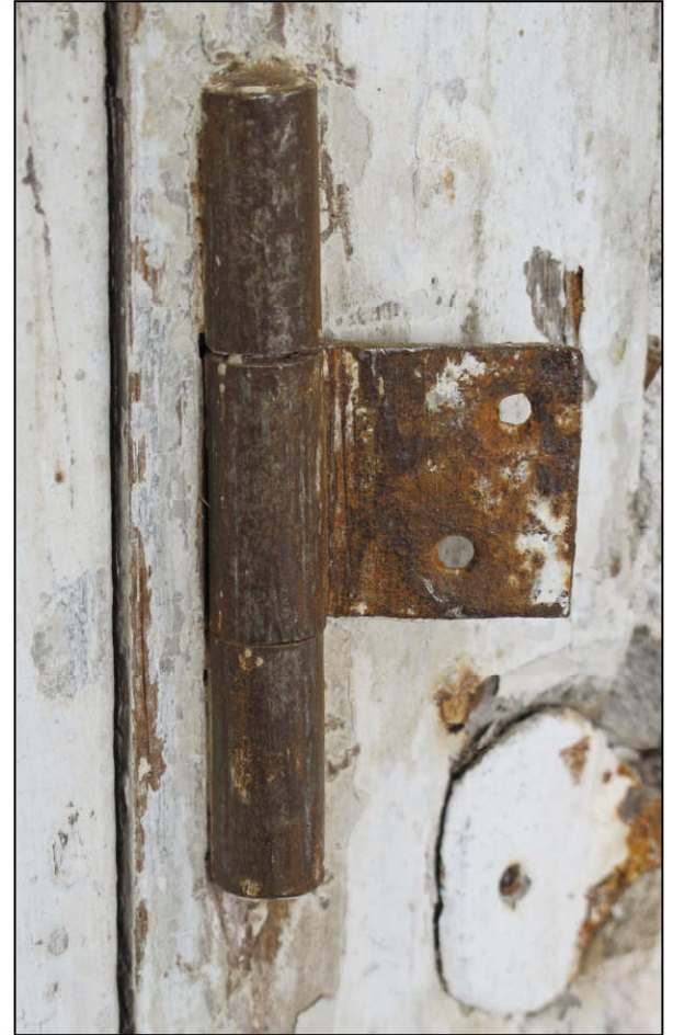
Fig. 7.3. Fiche (volet)
