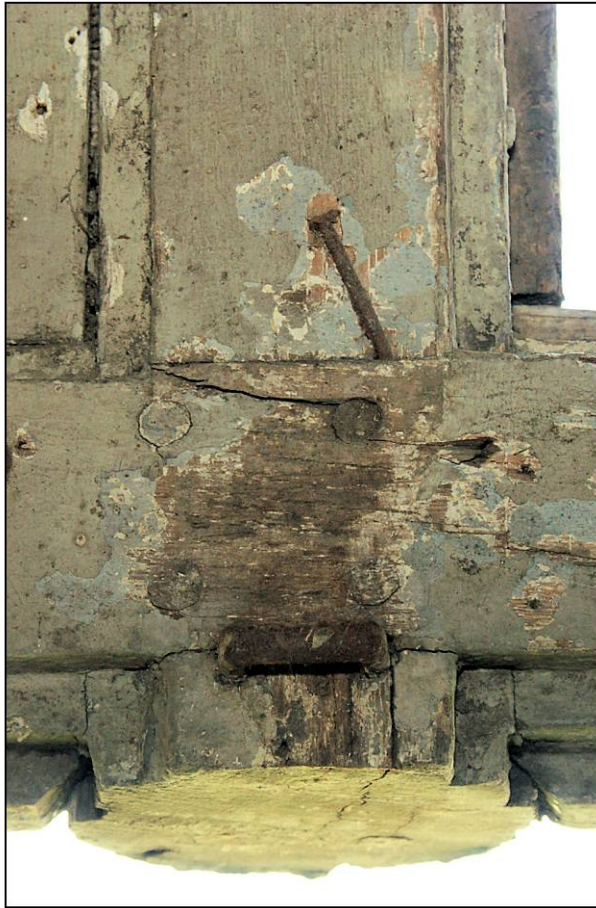
Fig. 2.2. Assemblage meneau / croisillon
