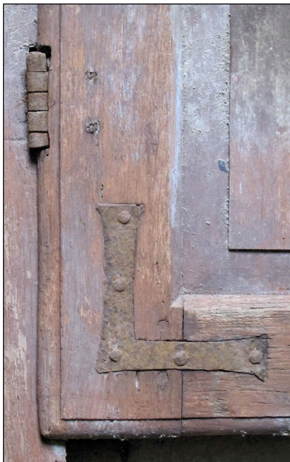
Fig. 5.3. Fiche à broche rivée et équerre
