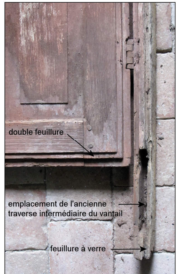
Fig. 5.5. Assemblage montant / traverse inter.
