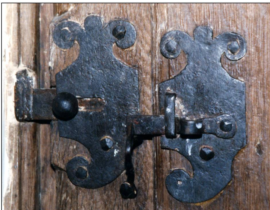
Fig. 4.7. Targette enclouonnée et loquet
