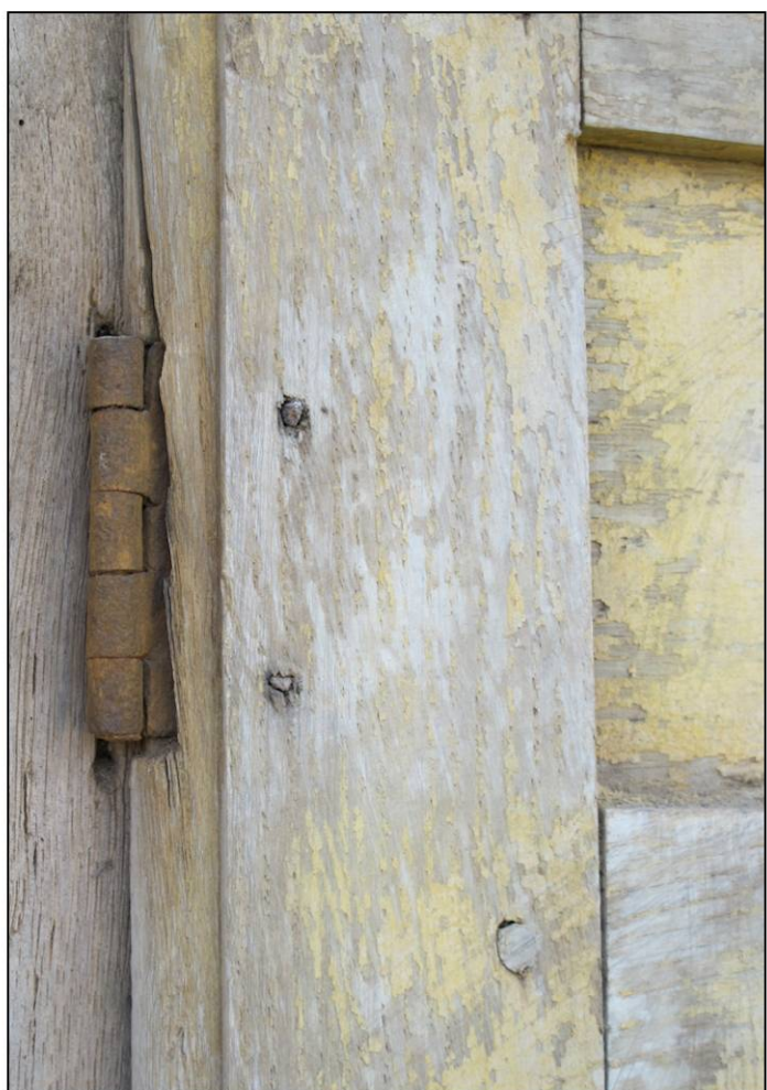
Fig. 1.3. Fiche à broche rivée
