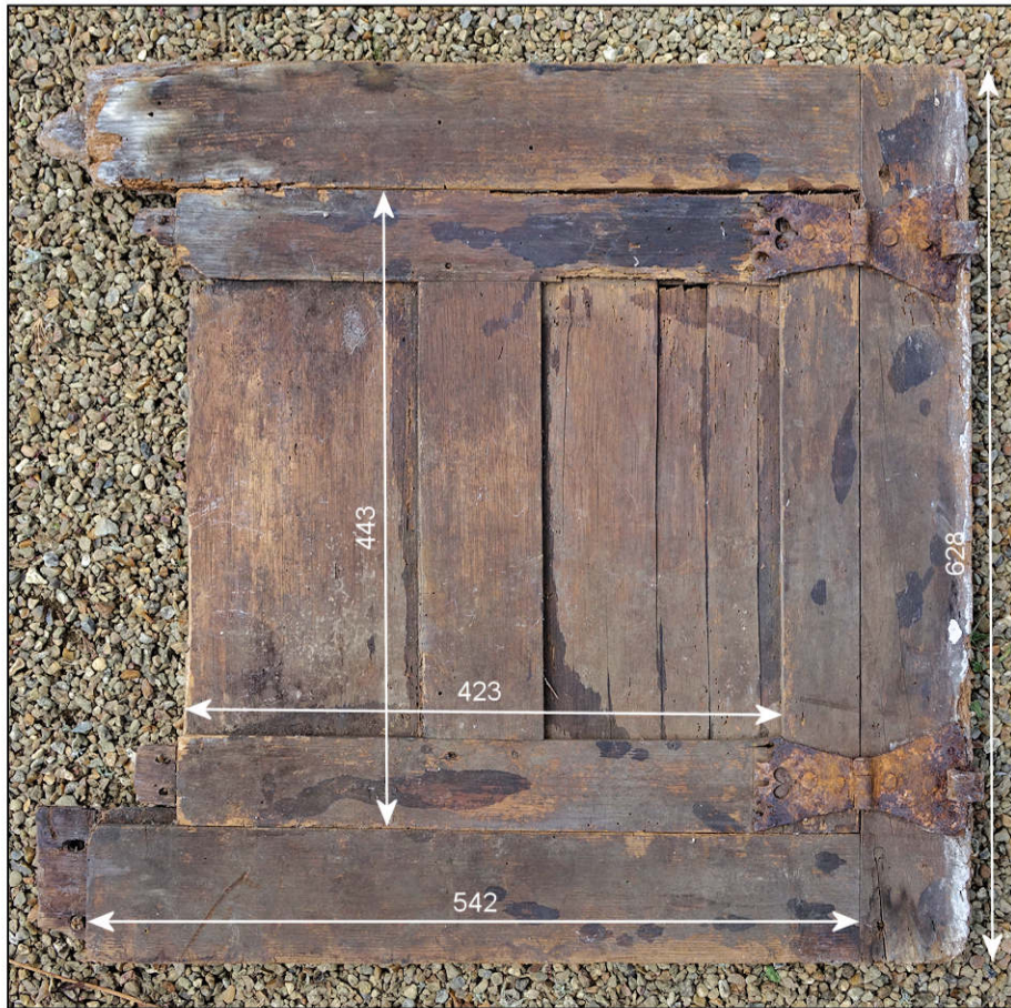
Fig. 5.1. Vue intérieure
